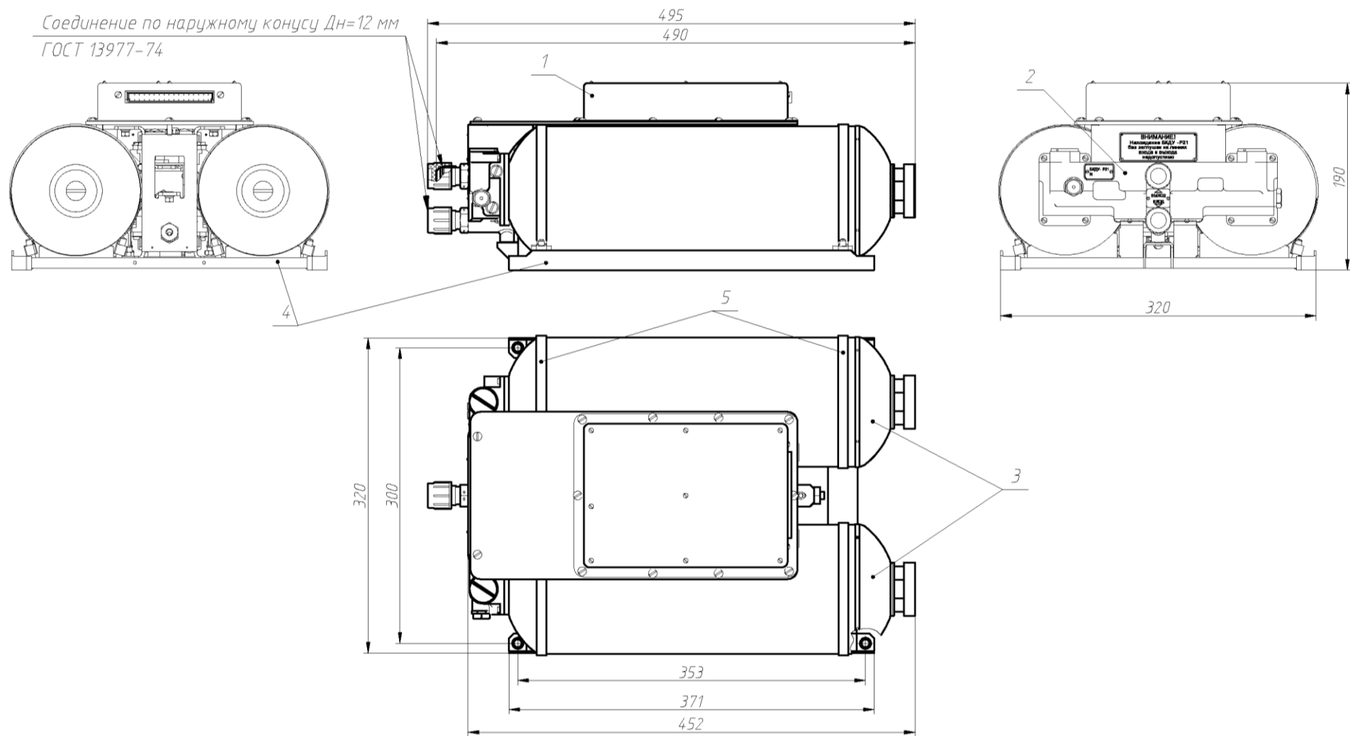
Рисунок 1. Установка бортовая кислорододобывающая.
