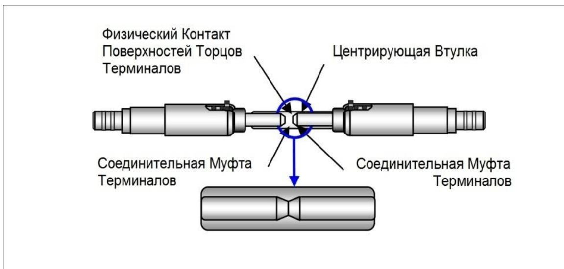
Рисунок 1 – Интерфейс и центровка оптоволоконных терминалов
