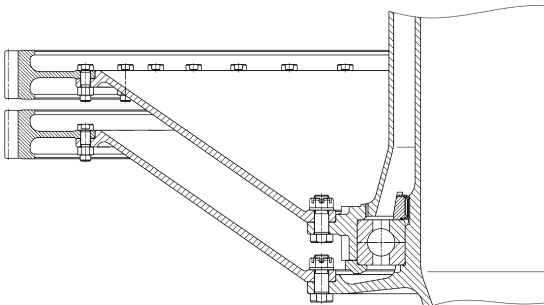
Рисунок 7 – Крепление зубчатых колес ( z=180 ) четвертой ступени редукции к валам несущих винтов
